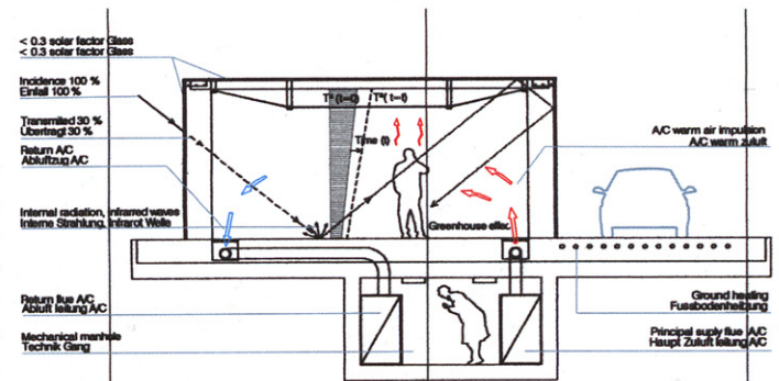
58 · SECCIÓN TRANSVERSAL DE LA RAMPA
